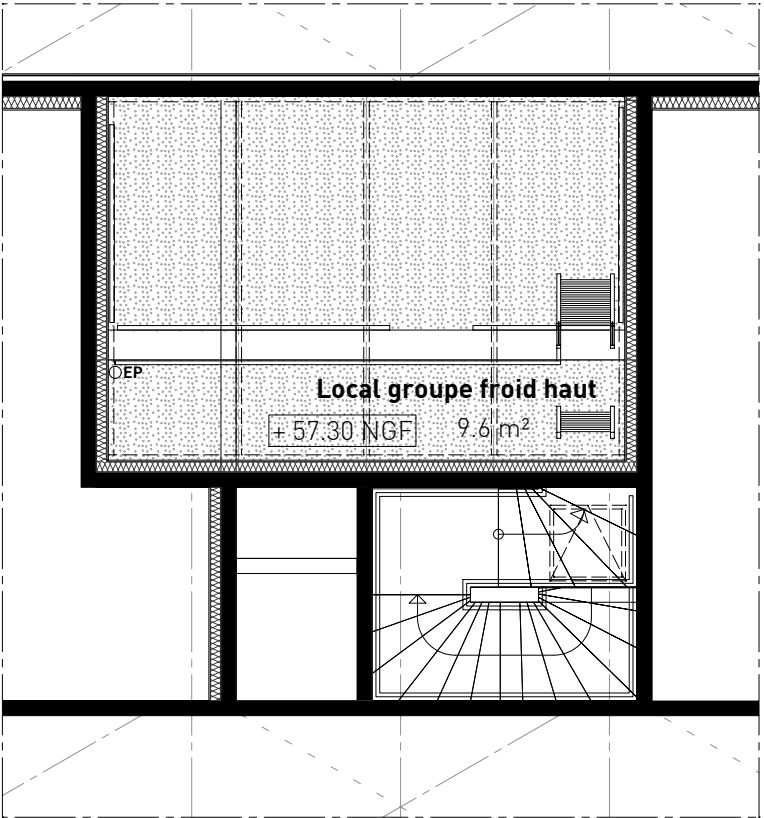
Plan R+2 - Local groupe froid
